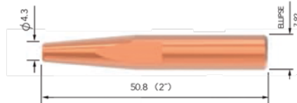
Punte di contatto BND - BND Contact Tips
